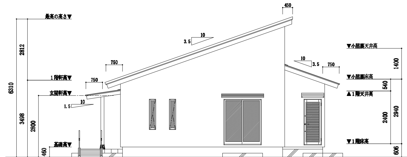
東立面図 S = 1 / 100
