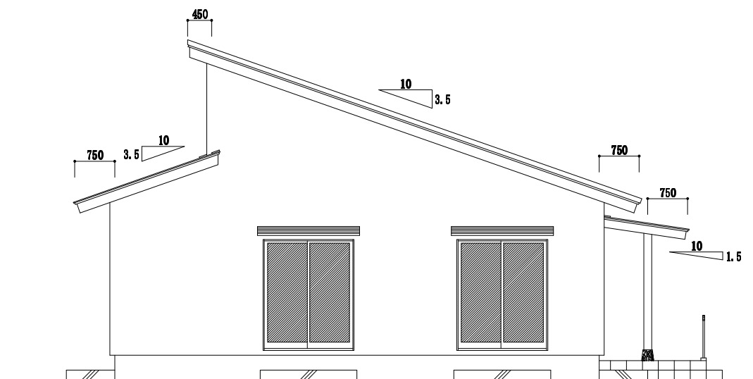
西立面図 S = 1 / 100
