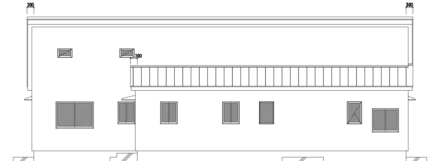
北立面図 S = 1 / 100
